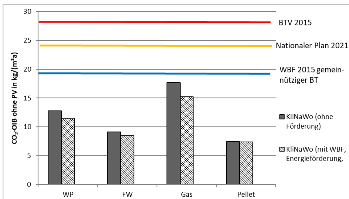
Abbildung 1: Kostenoptima der CO 2 -Emissionen nach OIB-RL 6 2011, differenziert nach Wärmeversorgungssystem – mit und ohne Berücksichtigung der Förderung.
