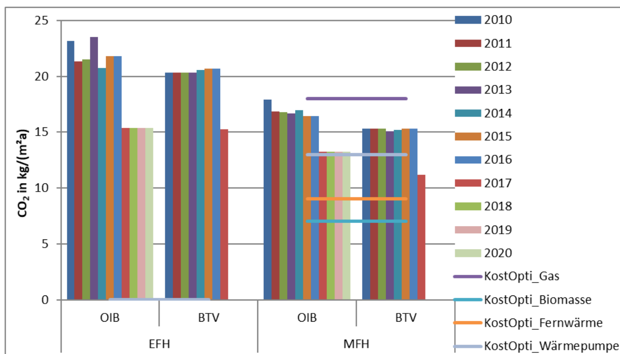
Abbildung 4: Spezifische CO 2 -Emissionen der Referenzgebäude gewichtet nach Energieträger für das Anforderungsniveau OIB-RL 6 und BTV. Zusätzlich ist das Kostenoptimum für MFH dargestellt (inklusive Haushaltsstrom).
