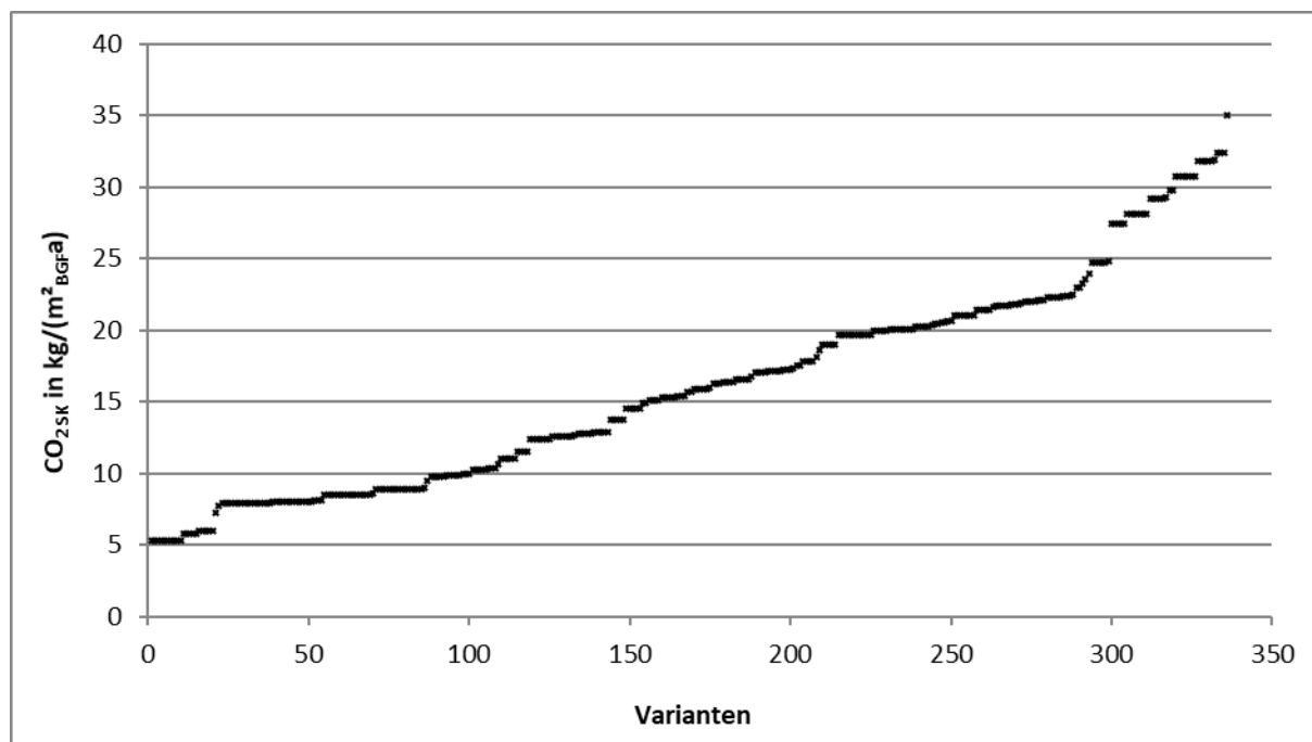
Abbildung 2: CO 2 -Emissionen der 336 untersuchten Varianten der Referenzgebäude (Punkte überlagern sich teilweise).
