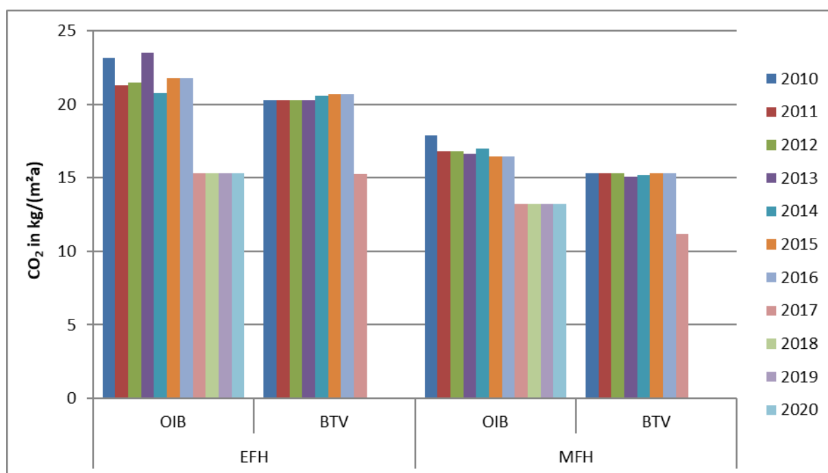
Abbildung 3: Spezifische CO 2 -Emissionen der Referenzgebäude gewichtet nach Energieträger für die Jahre 2010 bis 2020 getrennt nach Anforderungsniveau (inklusive Haushaltsstrom).
